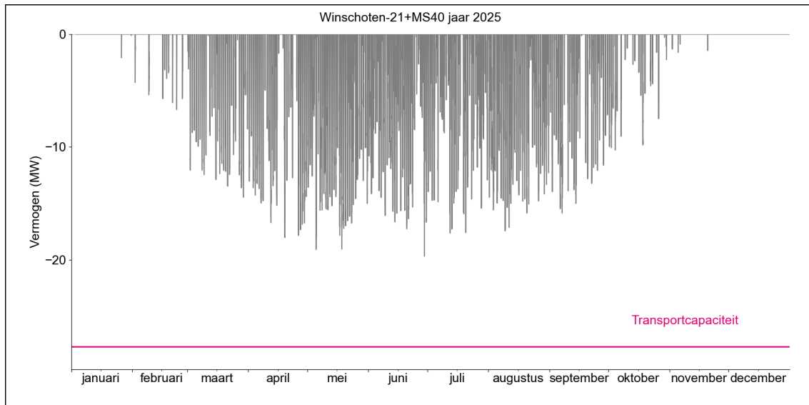
Figuur 2. Gerealiseerde transportbelasting voor invoeding op HS/MS-station Winschoten MS10-11+MS20-21+MS40 in 2025.
