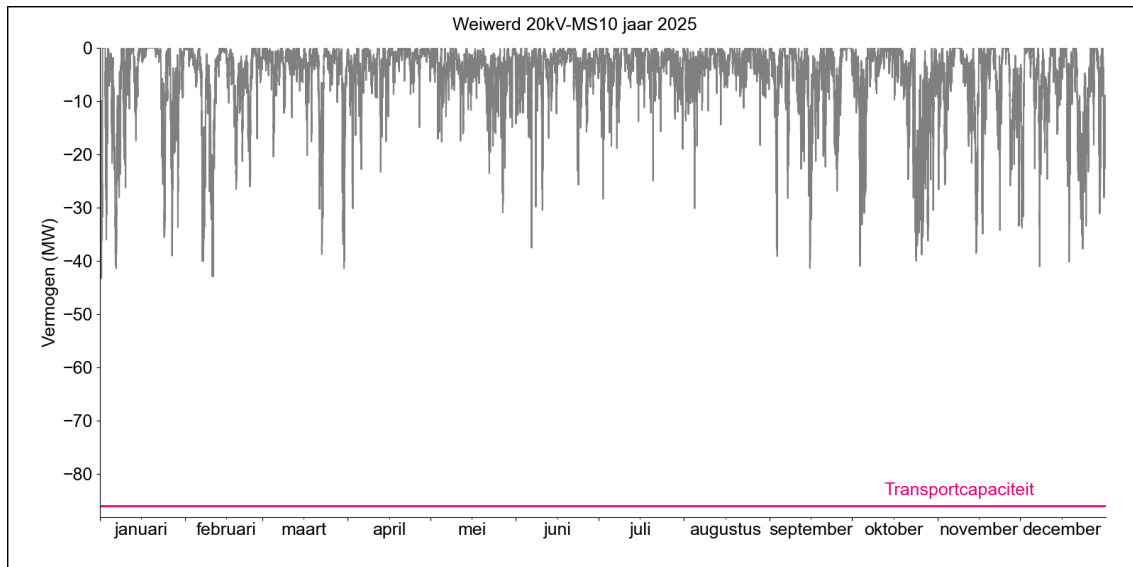
Figuur 2. Gerealiseerde transportbelasting voor invoeding op HS/MS-station Weiwerd MS10 + MS30 in 2025.
