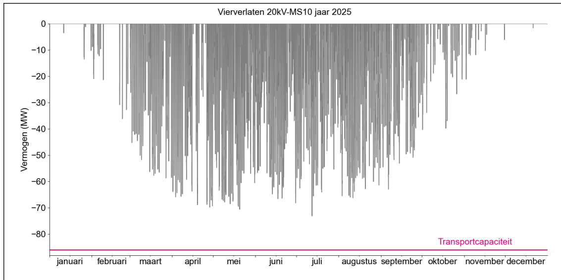
Figuur 2. Gerealiseerde transportbelasting voor invoeding op HS/MS-station Vierverlaten 20 kV MS10 in 2025.
