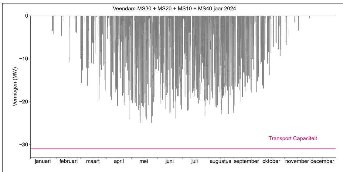
Figuur 2. Gerealiseerde transportbelasting voor invoeding op HS/MS-station Veendam MS30 + MS20 + MS10 + MS40 in 2024.
