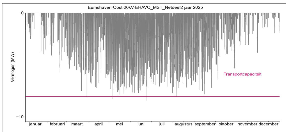
Figuur 2. Gerealiseerde transportbelasting voor invoeding op netdeel Eemshaven-Oost 20 kV EHAVO_MST_Netdeel2 in 2025.
