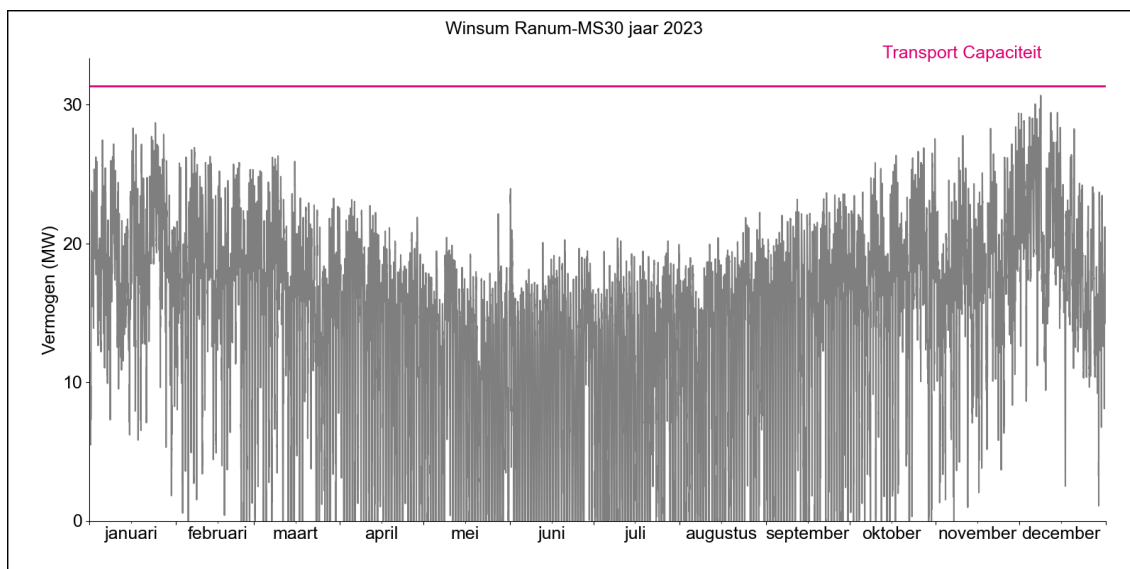
Figuur 2. Gerealiseerde transportbelasting voor afname op HS/MS-station Winsum Ranum MS30 in 2023.
