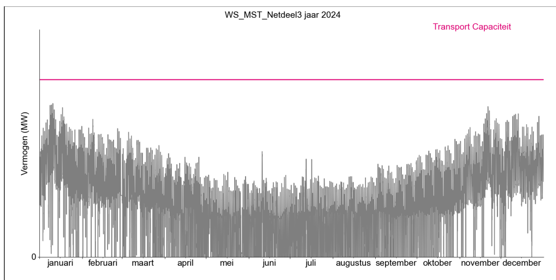
Figuur 2. Gerealiseerde transportbelasting voor afname op netdeel Winschoten WS_MST_Netdeel3 in 2024.
