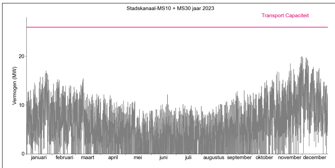
Figuur 2. Gerealiseerde transportbelasting voor afname op HS/MS-station Stadskanaal MS10 + MS30 in 2023.
