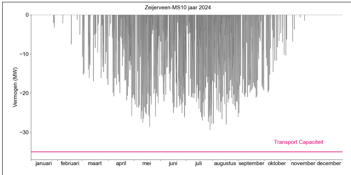
Figuur 2. Gerealiseerde transportbelasting voor invoeding op HS/MS-station Zeijerveen MS10 in 2024.
