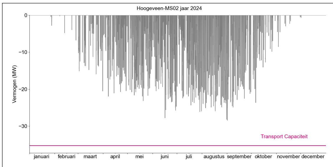
Figuur 2. Gerealiseerde transportbelasting voor invoeding op HS/MS-station Hoogeveen MS02 in 2024.
