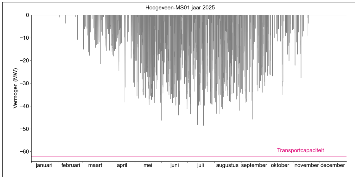
Figuur 2. Gerealiseerde transportbelasting voor invoeding op HS/MS-station Hoogeveen MS01 in 2025.
