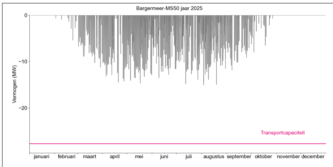
Figuur 2. Gerealiseerde transportbelasting voor invoeding op HS/MS-station Bargermeer MS50 in 2025.
