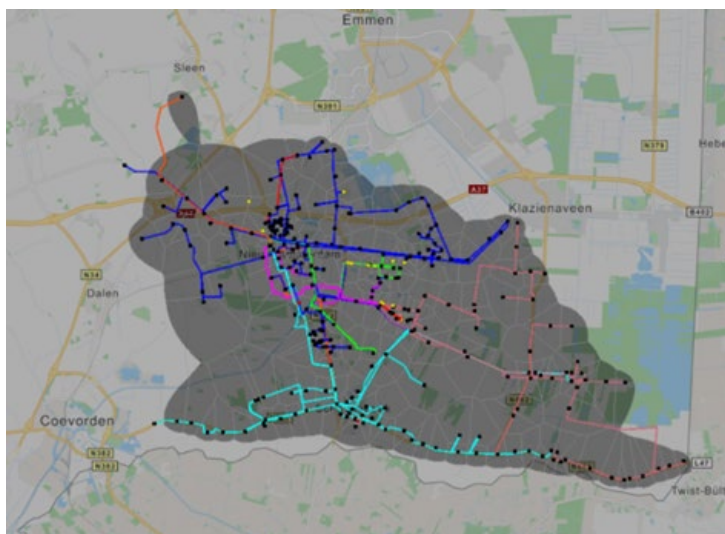
Figuur 1. Geografische indicatie van het voorzieningsgebied van HS/MS-station Veenoord MS01.
