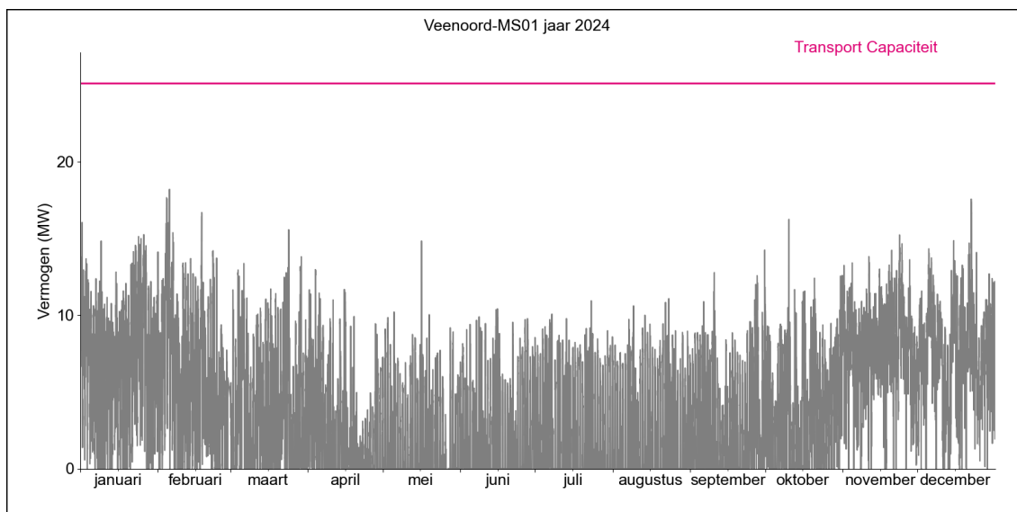
Figuur 2. Gerealiseerde transportbelasting voor afname op HS/MS-station Veenoord MS01 in 2024.
