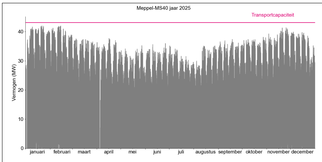
Figuur 2. Gerealiseerde transportbelasting voor afname op HS/MS-station Meppel MS40 in 2025.
