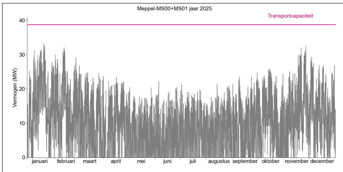
Figuur 2. Gerealiseerde transportbelasting voor afname op HS/MS-station Meppel MS00 + MS01 in 2025.
