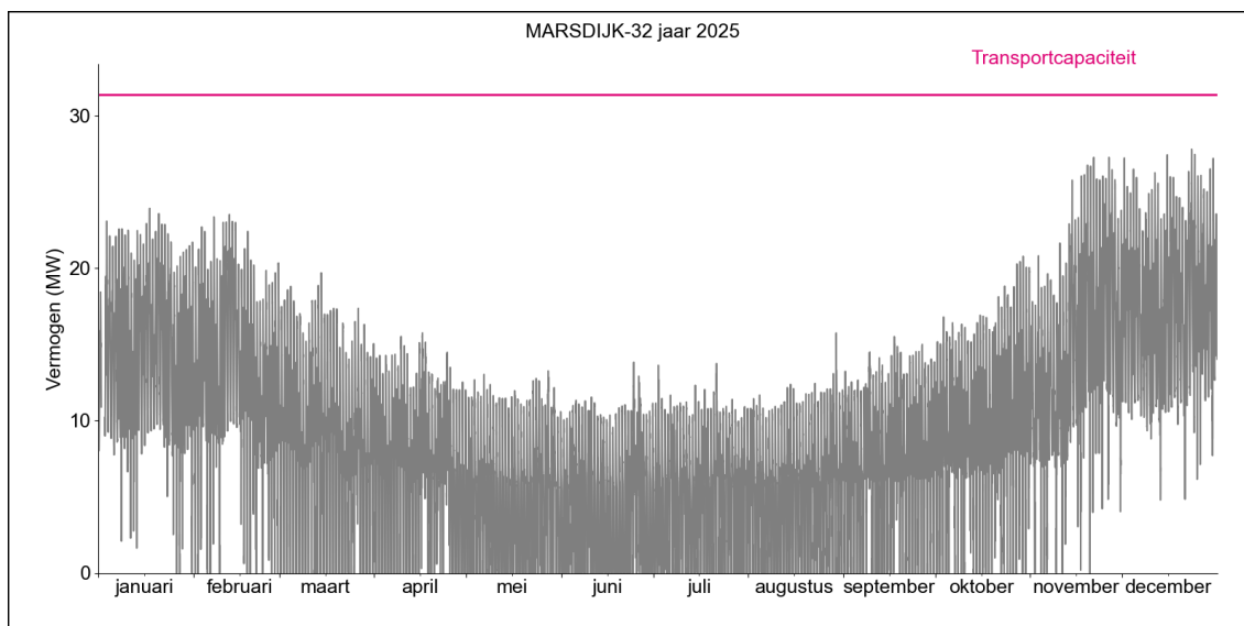
Figuur 2. Gerealiseerde transportbelasting voor afname op HS/MS-station Marsdijk Rail 12+22+32 in 2025.
