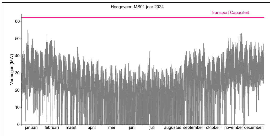
Figuur 2. Gerealiseerde transportbelasting voor afname op HS/MS-station Hoogeveen MS01 in 2024.
