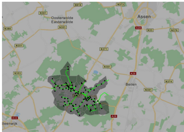
Figuur 1. Geografische indicatie van het voorzieningsgebied van netdeel Beilen BL_MST_Netdeel1.
