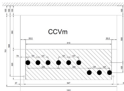
Afbeelding 8: vloerplan ABB Safepus-Air CCVm-DCO
