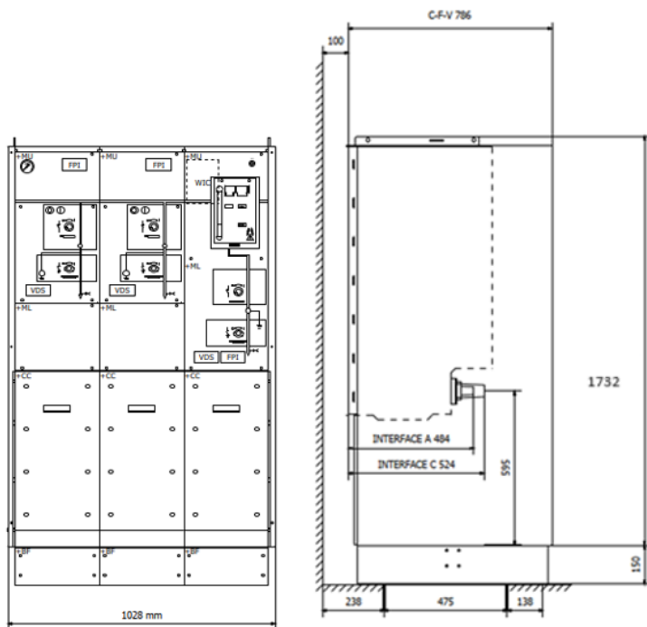
Afbeelding 7: ABB Safepus-Air CCVm-DCO
