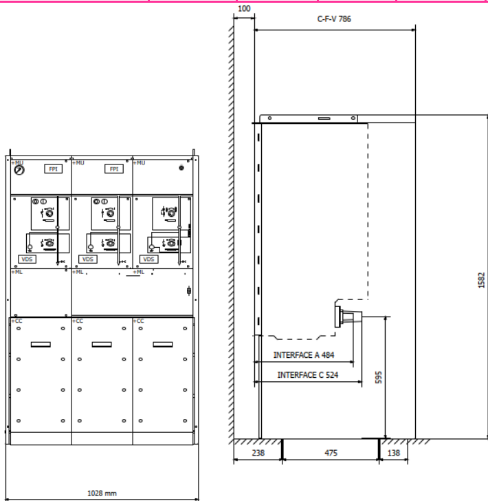
Afbeelding 5: ABB Safepus CCF-Air
