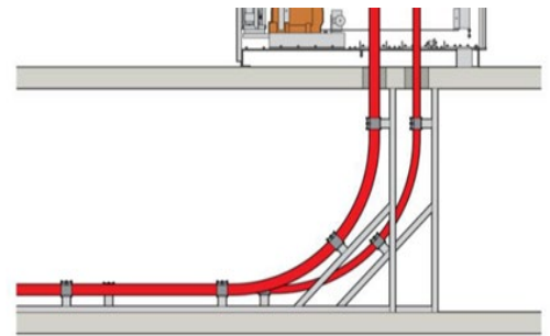
Afbeelding 4: kelder met kabelopvoerconstructie
